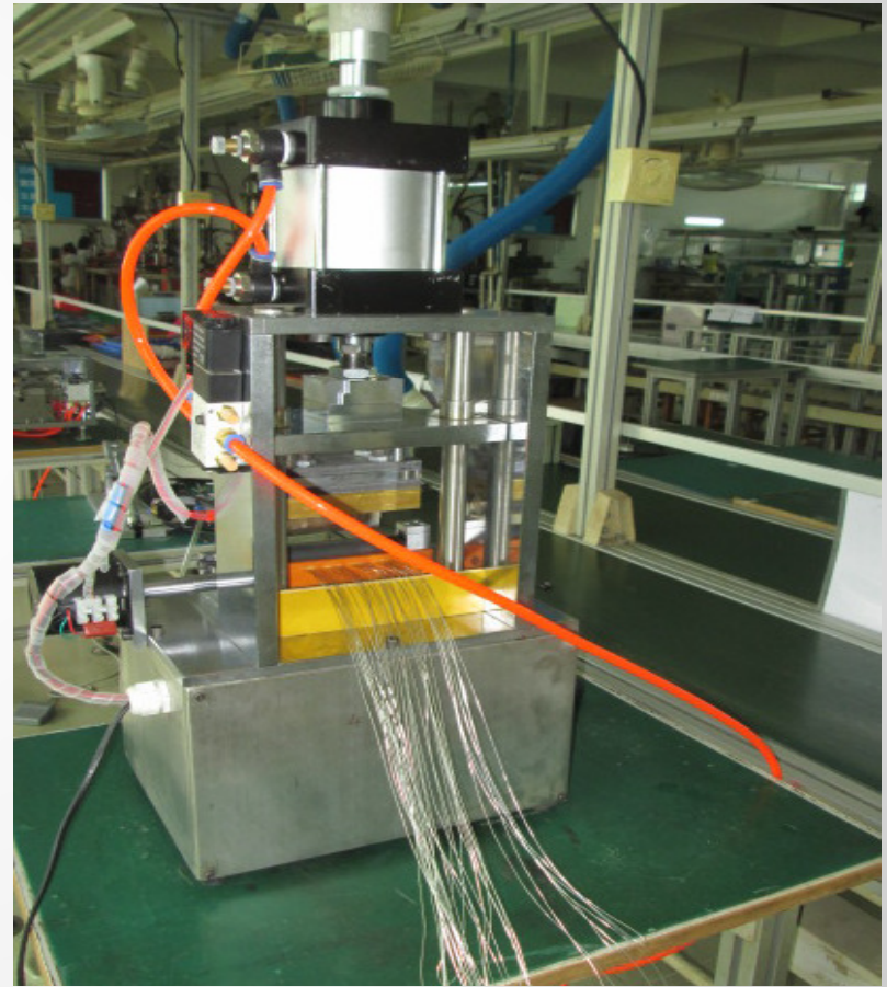
HDMI上錫機
